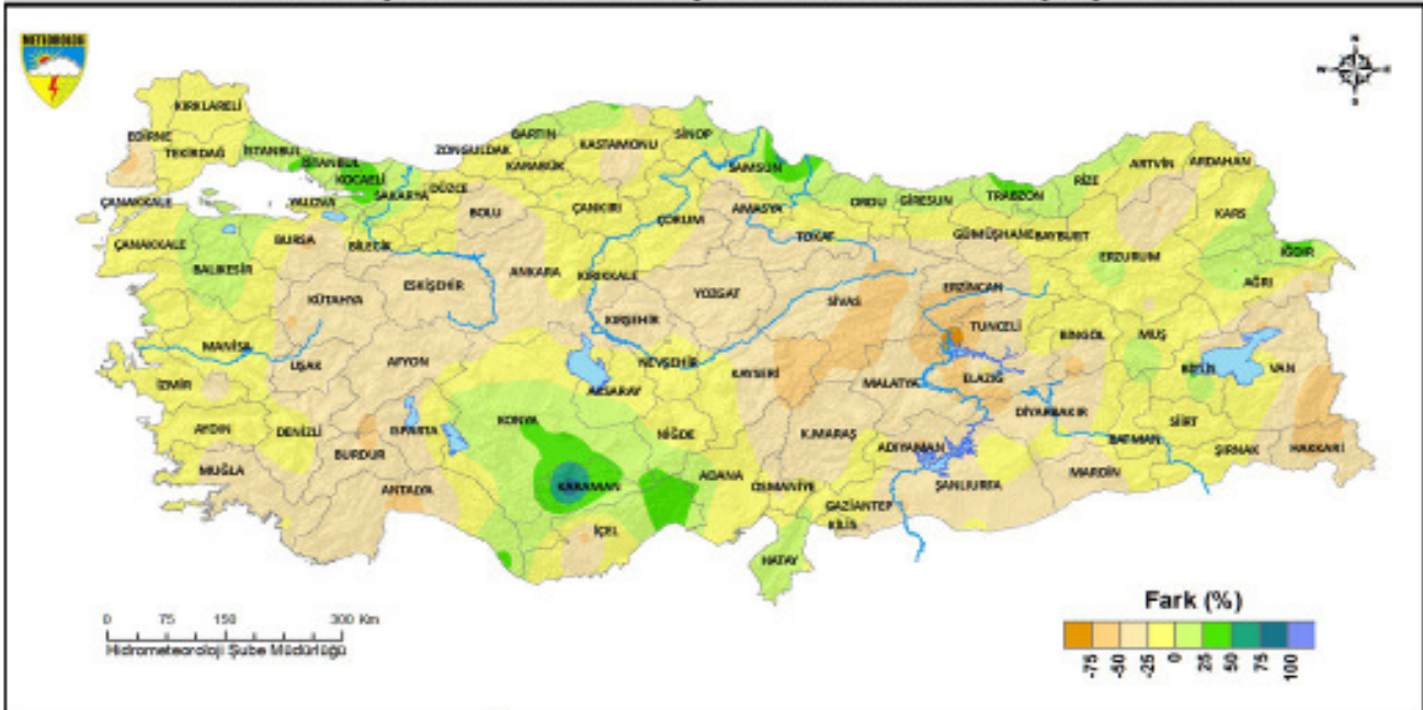
Şekil 3. 2017 Kış Mevsimi Alansal Yağışların Normali İle Karşılaştırılması
